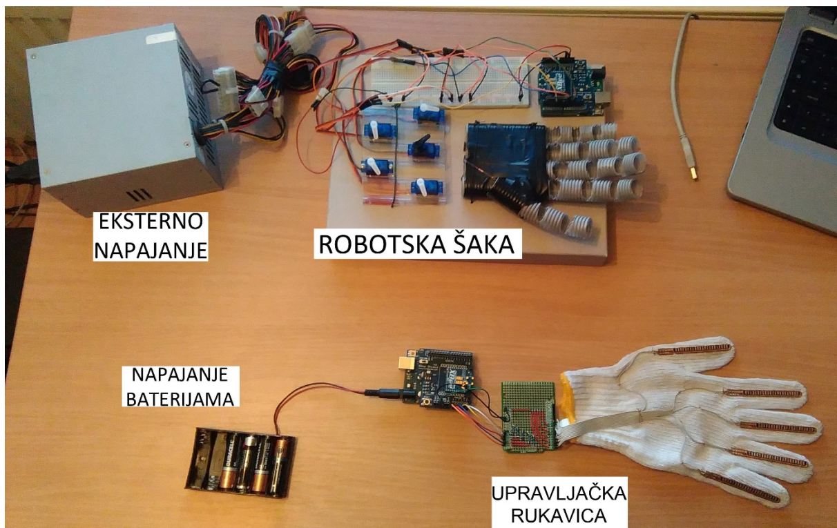
Slika 2. Sustav bežične animatroničke šake
