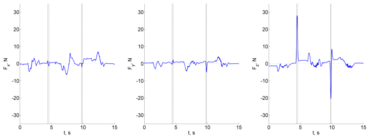
Slika 5.12. Komponente sile.
