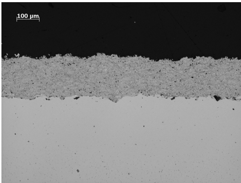
Slika 25. SEM slika poprečnog presjeka uzorka naštrcanog \text{Cr}_3\text{C}_2 prevlakom
