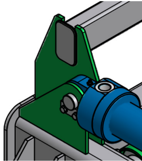
Slika 50. Držać cilindra
