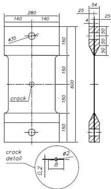
Slika 1. Uzorak ploče sa središnjom pukotinom P1 Figure 1. Centrally notched plate specimen P1
