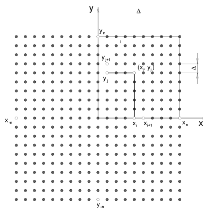
Figure 8. Stochastic lattice Slika 8. Stohastička rešetka
