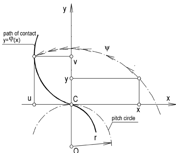
Figure 7. Two dimensional transformation Slika 7. Dvodimenzijaska transformacija
