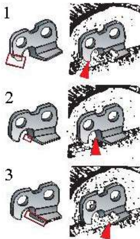
Slika 22. Princip rada reznog zuba[9]
