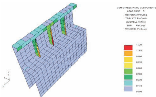
Slika 8 Omjer stvarnih i dopuštenih napreznja na pražnici grotla
