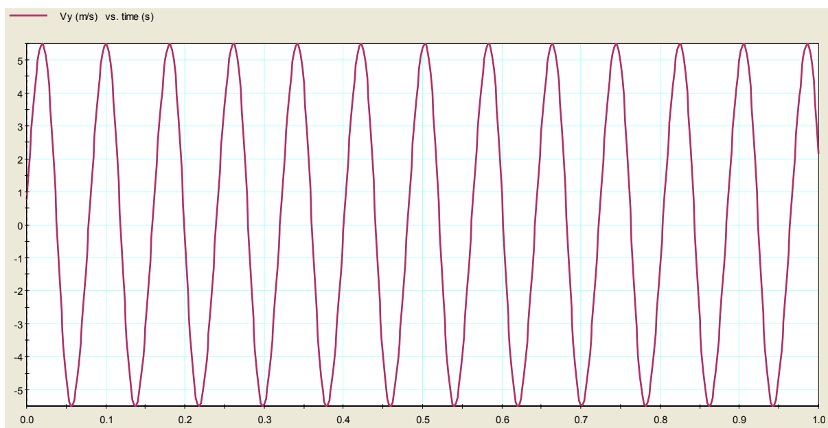
Slika 21. Brzina stapa 4
