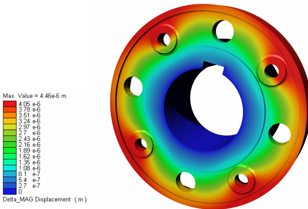
Slika 79. Raspodjela pomaka
