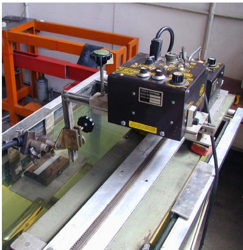
Slika 3.1 Sustav za automatsko zavarivanje Bugo Systems BUGO-5300 postavljen na laboratorijski bazen
