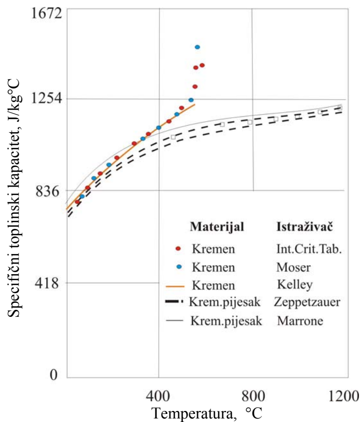
Slika 4.45 Specifični toplinski kapacitet kristala kremenata i kremenog pijeska [31]
