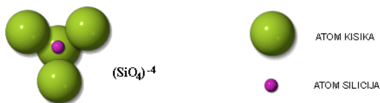
Slika 3.2 Silikatni tetraedar
