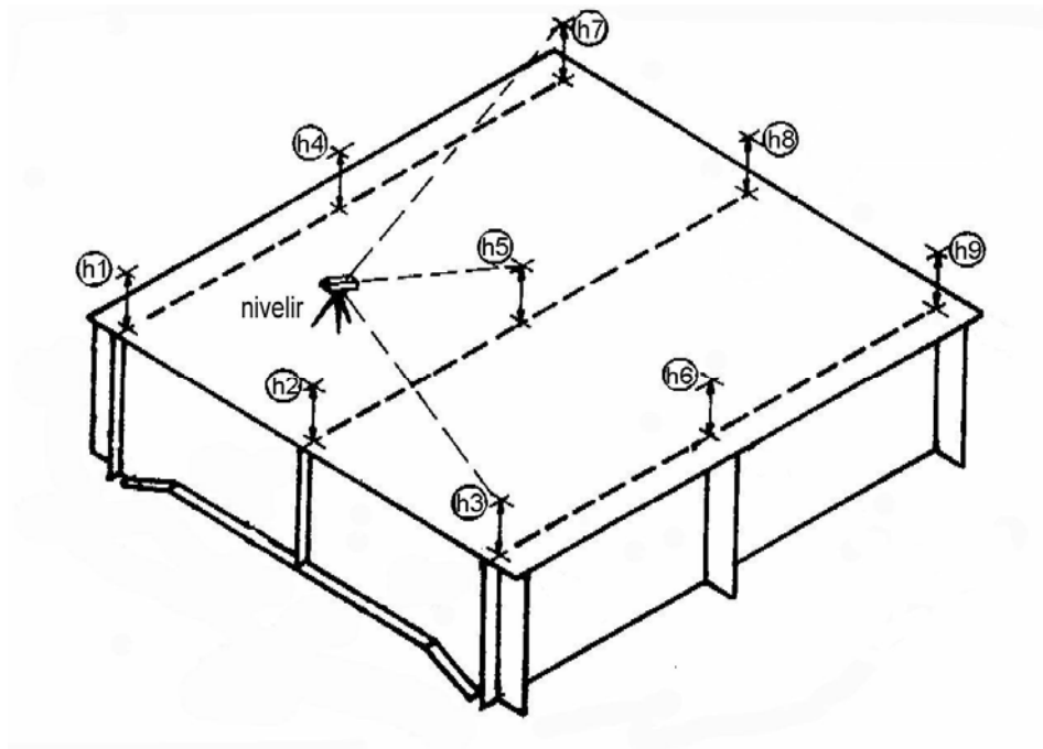
Slika 11: Kontrola ravnine oploćenja sekcije
