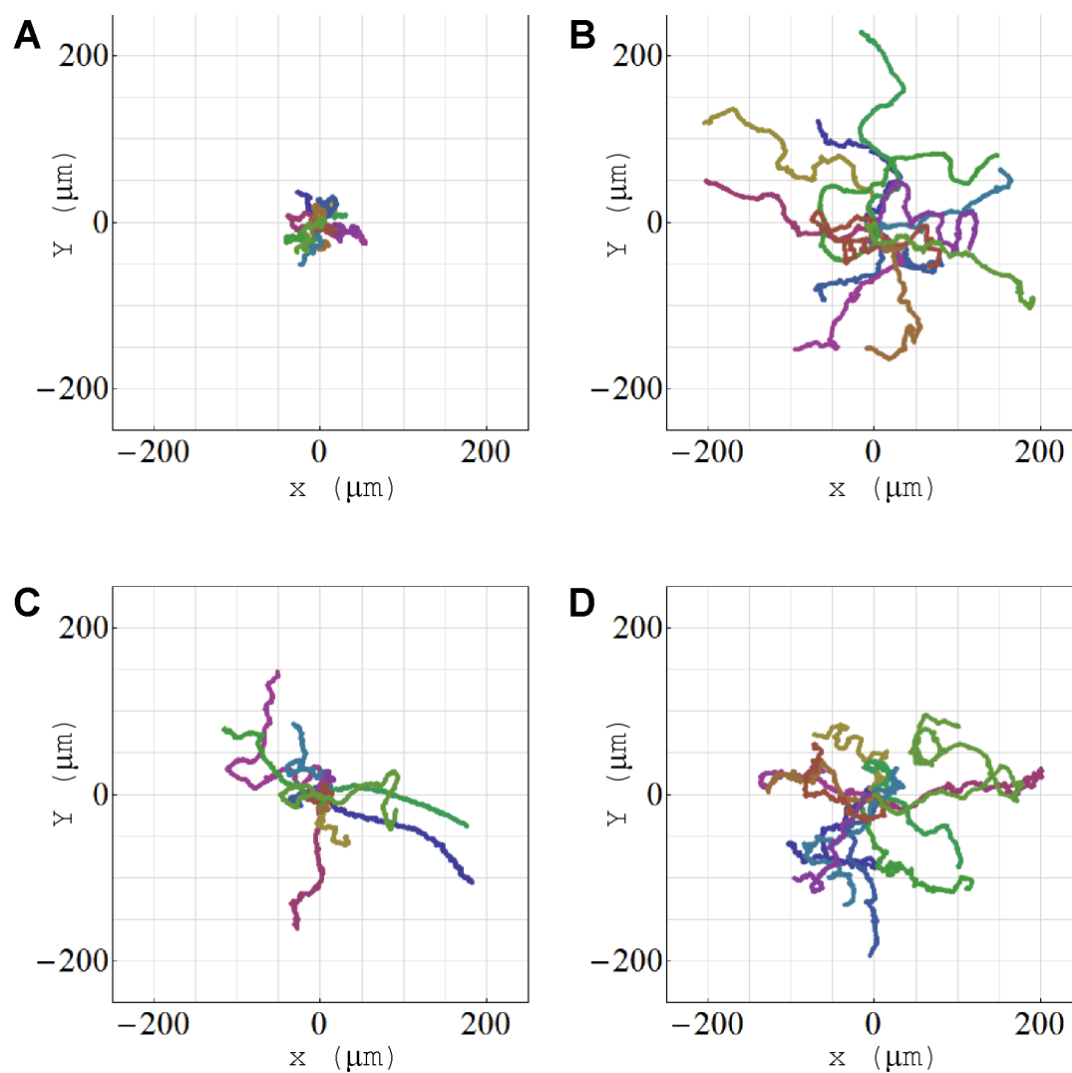
Slika 3.3. Karakteristične trajektorije stanica četiri različitih populacija D. discoideum praćenih tijekom 40 min: (A) vegetativnih AX2, (B) agregacijski kompetentnih AX2, (C) vegetativnih CI/CI' i (D) agregacijski kompetentnih CI/CI' stanica. Za svaku populaciju prikazano je 12 trajektorija.
