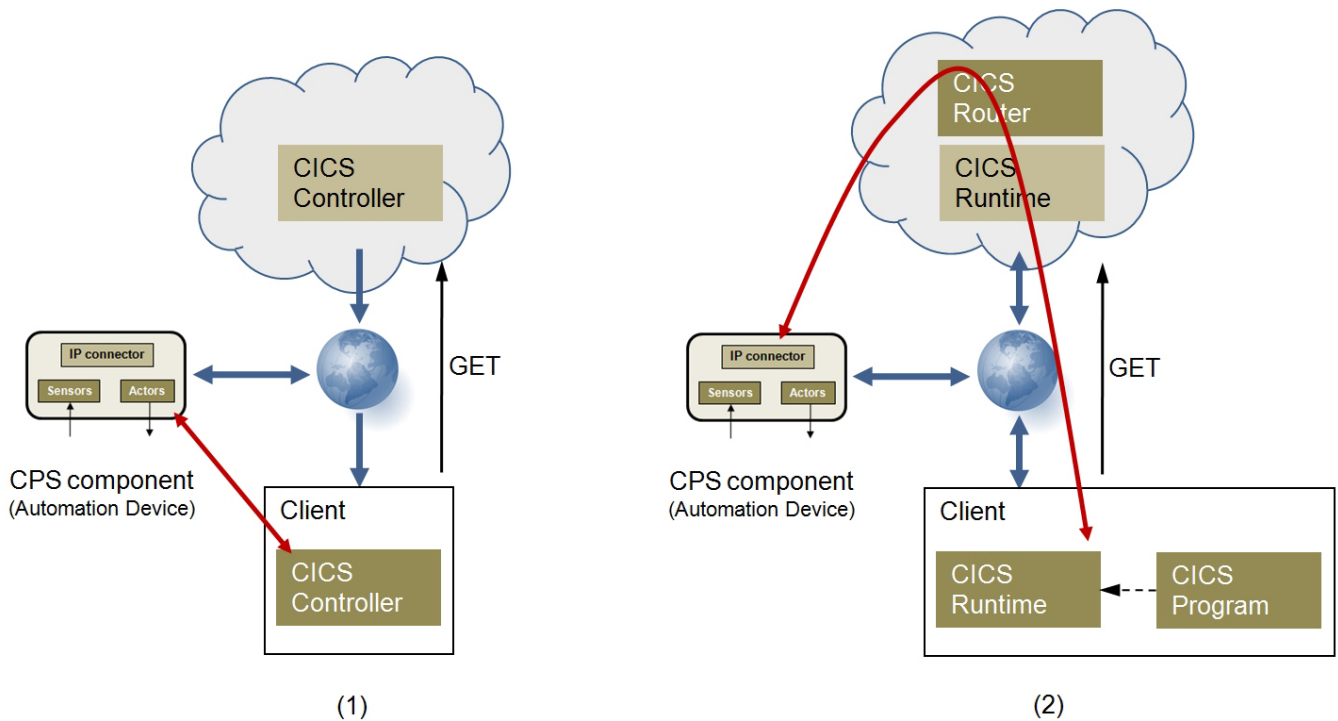
Abb. 7 Komponentenstruktur und Kommunikationswege für client-basierte CICS-Lösungen
