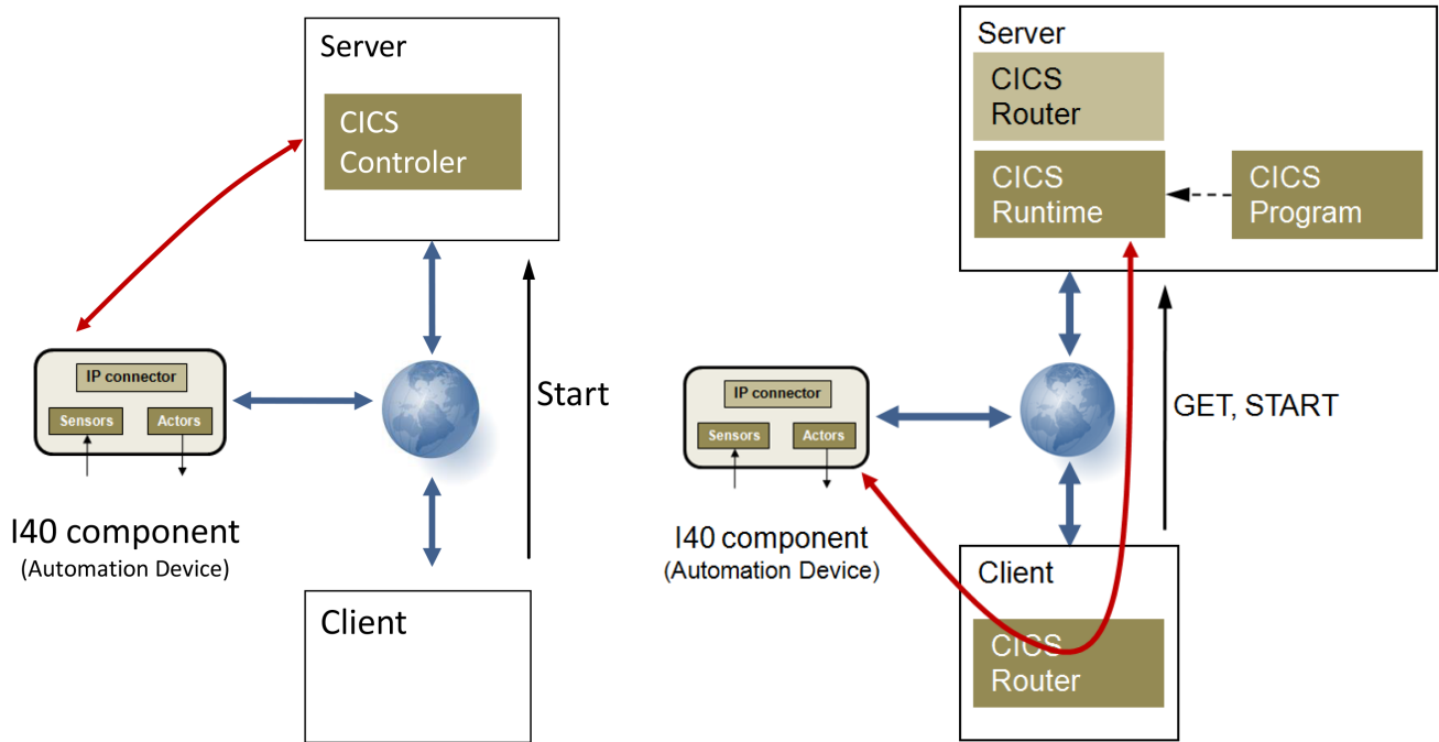
Abb. 6 Komponentenstruktur und Kommunikationswege für server-basierte CICS-Lösungen
