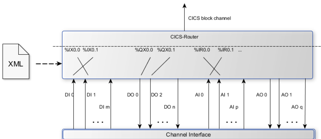
Abb. 8 CICS-Router
