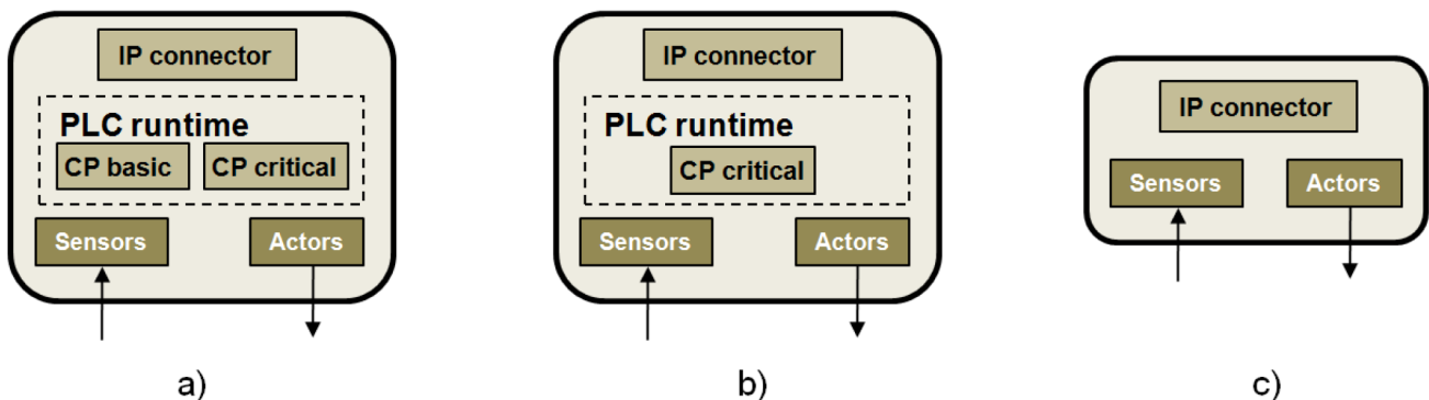
Abb. 5 Evolution einer Industriesteuerung (SPS) als CPS-Komponente
