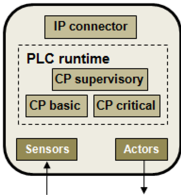
Abb. 4 Struktur einer SPS als CPS-Komponente
