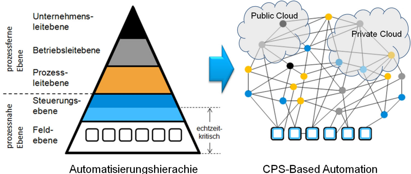
Abb. 1 Auflösung der klassischen Automatisierungspyramide und Verlagerung von Funktionen als Dienste in eine Cloud
