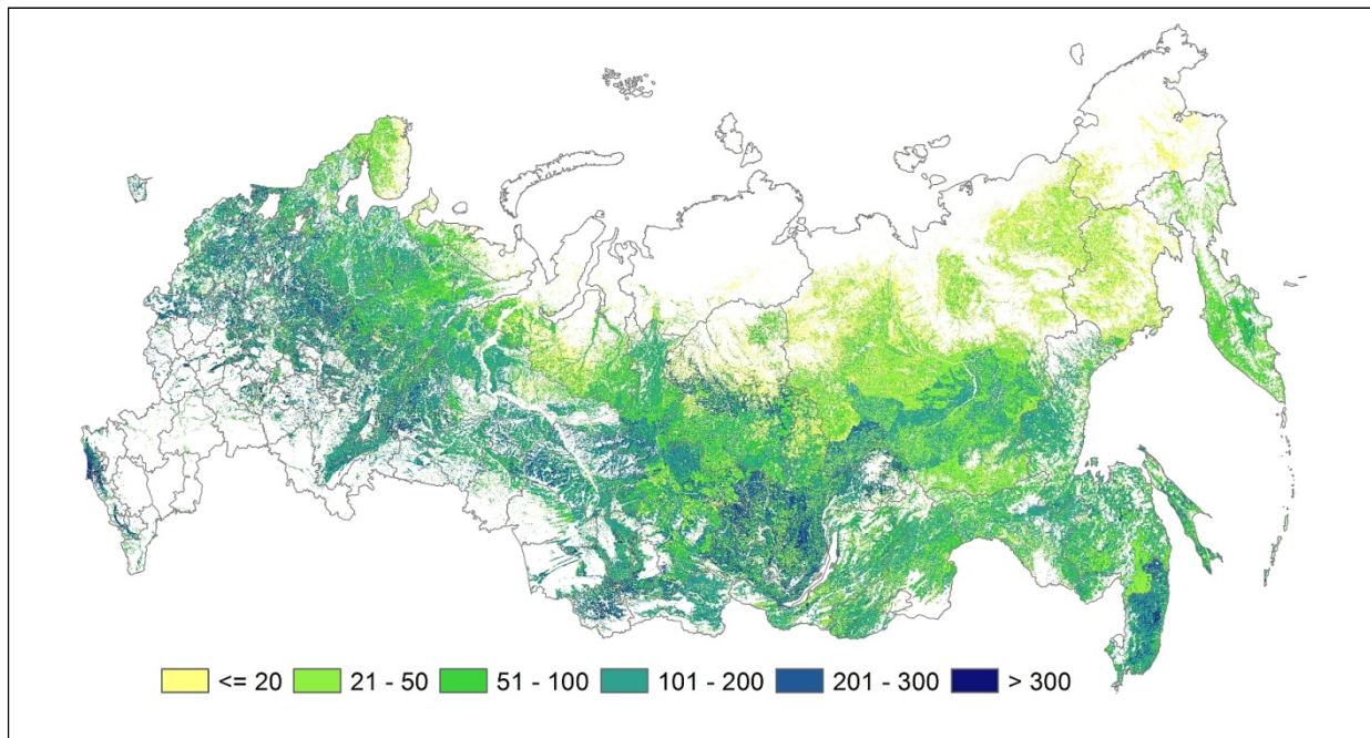
Рис.1. Средние запасы лесов России ( \text{м}^3 \text{га}^{-1} )
