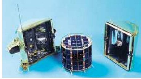
Fig. 1: Hopping robot MINERVA.
