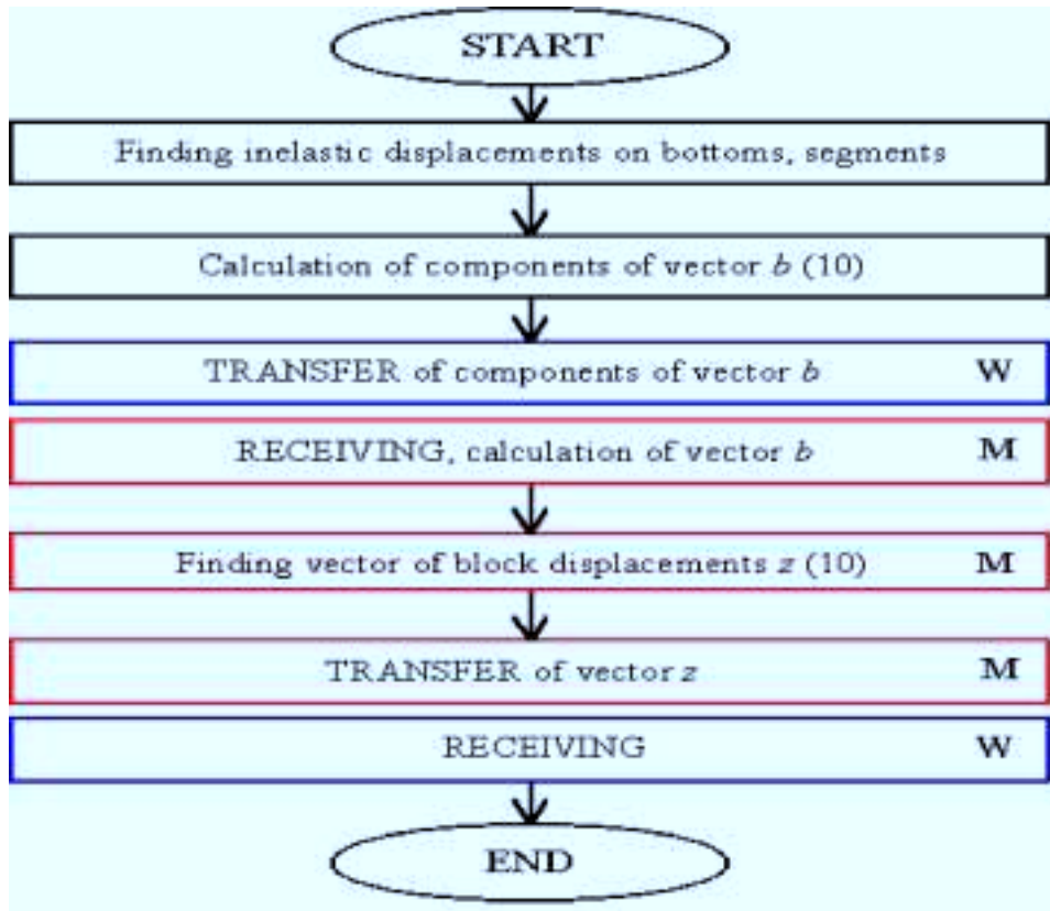
Fig. 4. Procedure CALC
