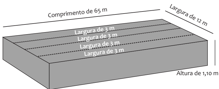
Figura 4. Desenho esquemático das dimensões da estação de compostagem com quatro leiras com largura de 3 m, medindo 65 m de comprimento e 12 m de largura total e 1,10 m de altura.
