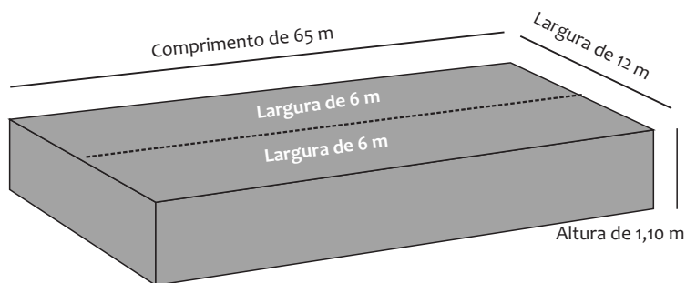
Figura 3. Desenho esquemático das dimensões da unidade de compostagem com duas leiras com largura de 6 m, medindo 65 m de comprimento e 12 m de largura total e 1,10 m de altura.
