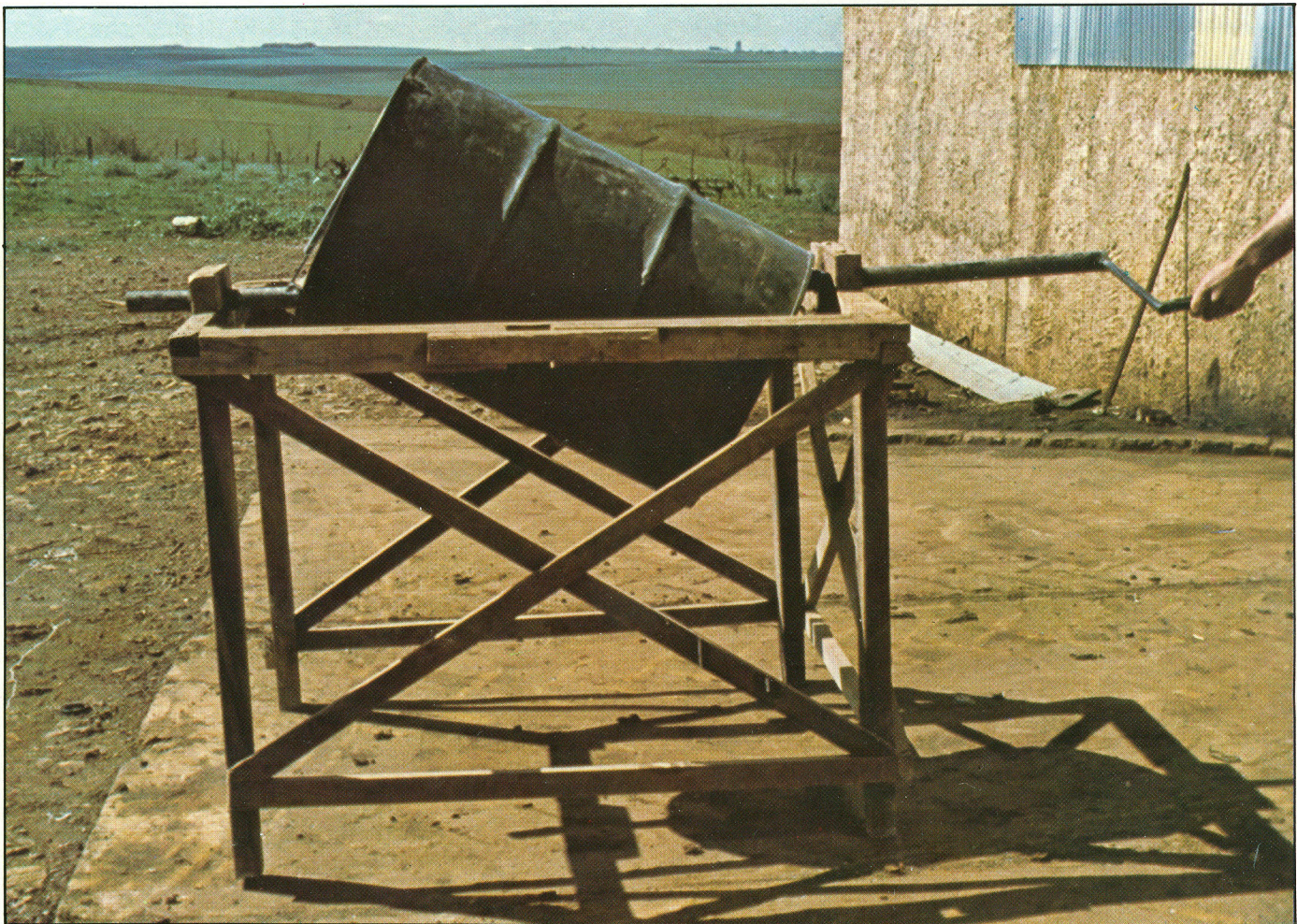
Figura 20. Tambor rotativo empregado no tratamento de sementes com fungicidas.
