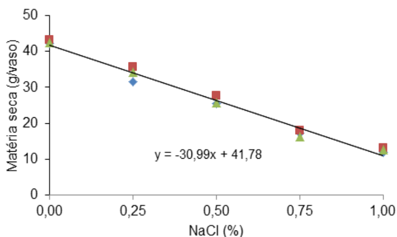
Figura 2. Produção de matéria seca (g) da parte aérea do arroz em função do nível de sal na água de irrigação. Avaliação realizada na diferenciação da panícula. Dados médios de cinco genótipos. Safra 2011/2012. Embrapa Clima Temperado, Pelotas, RS.
