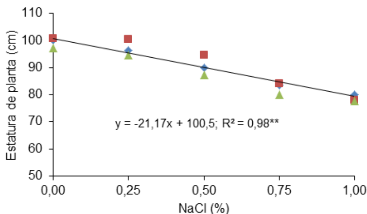
Figura 1. Estatura de planta (cm) arroz em função do nível de sal na água de irrigação. Avaliação realizada na diferenciação da panícula. Dados médios de cinco genótipos. Safra 2011/2012. Embrapa Clima Temperado, Pelotas, RS.
