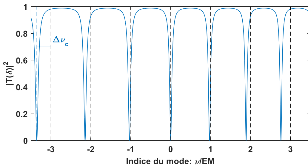
Fig 7. Structure modale d'un résonateur optique en régime de dispersion normale. L'espacement modal du résonateur diminue avec la fréquence en régime de dispersion normale.
