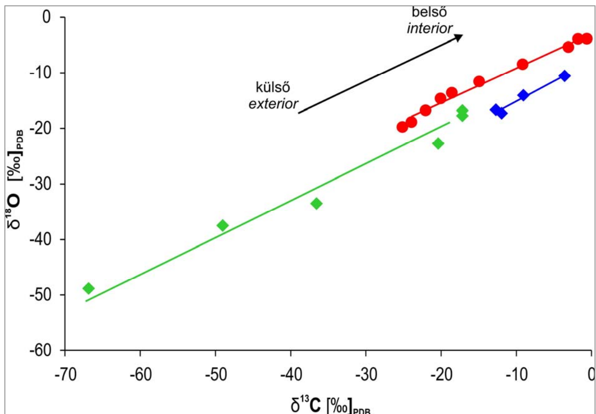
10. ábra: A homoródkarácsonyfalvai habarcs minták stabilizotópos összetétele (kék), összehasonlításként Kosednar-Legenstein et al. 2008 közleményéből római kori habarcs (piros) és laborkísérletből származó habarcs (zöld) stabilizotópos összetétele a külső szélétől a belseje felé.
