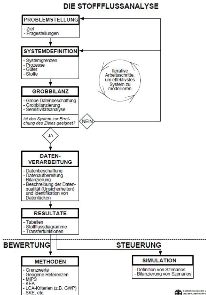
Abbildung 9: Stoffflussanalyse (Quelle: ÖWAV 2003:16)
