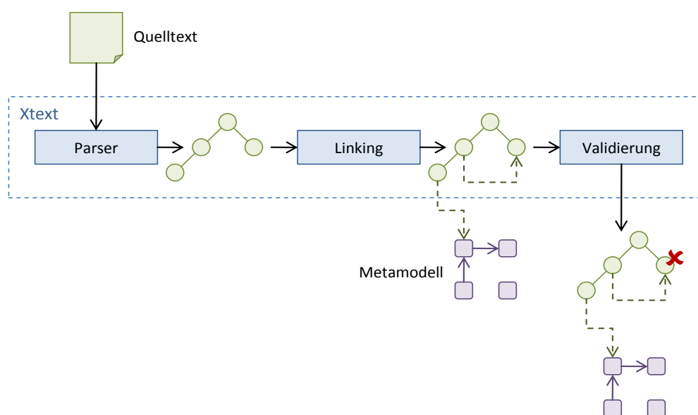
Abbildung 25: Die drei Phasen bei der Erzeugung eines aufgelösten und validierten Modells aus einer Quelldatei
