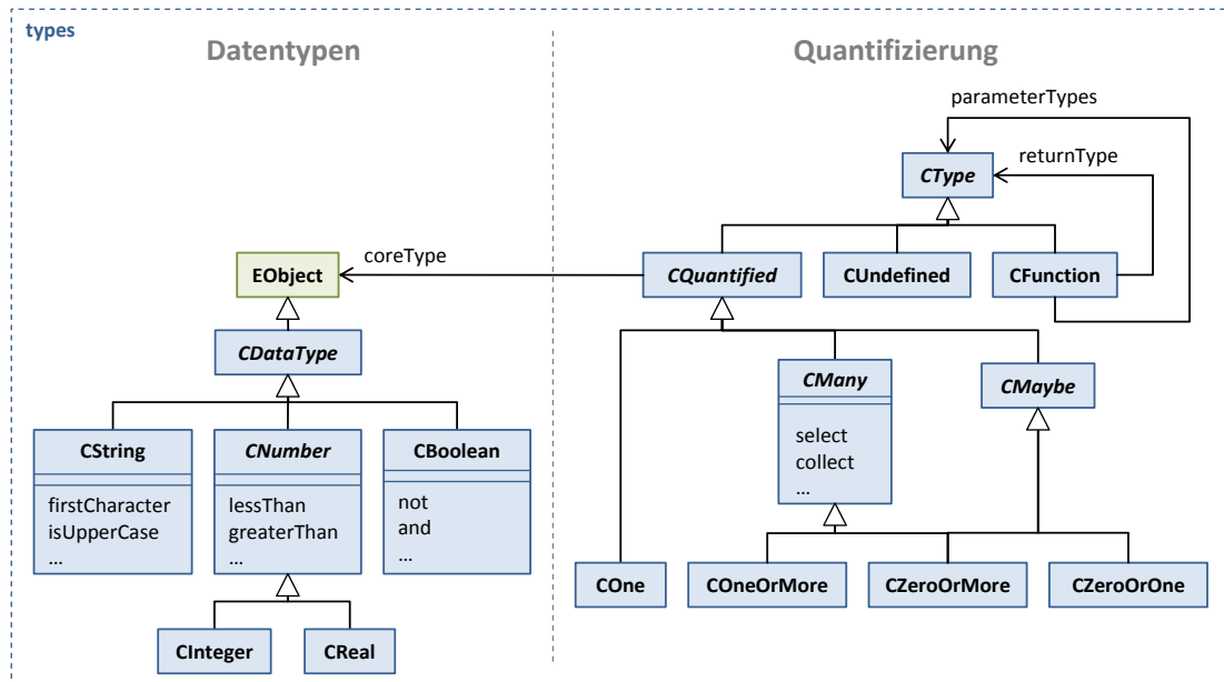
Abbildung 20: Semantisches Modell der Typen in LMMC
