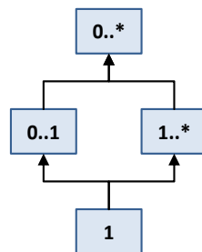
Abbildung 21: Ordnung der Multiplizitäten auf Basis der Teilmengenrelation
