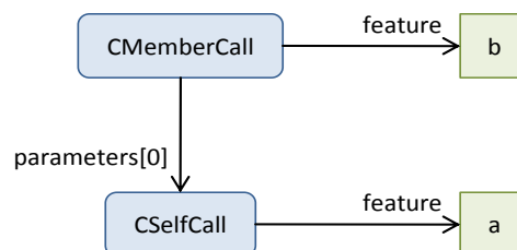
Abbildung 19: Instanz des semantischen Modells für den Ausdruck „a.b“
