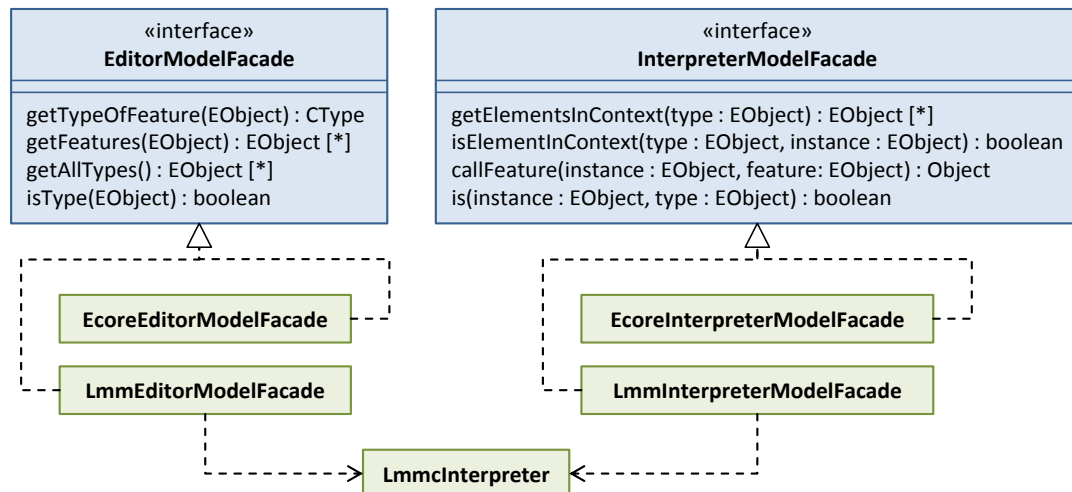
Abbildung 23: Implementierung der beiden Modellfassaden für Ecore und LMM
