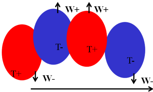
Abbildung 2: Schematische Darstellung warmer (T+) und kalter (T-) Turbulenzelemente. Durch die Verbindung mit einer aufwärtsgerichteten vertikalen Windkomponente (W+) oder einer abwärtsgerichteten vertikalen Windkomponente (W-) entsteht im turbulenten Windfeld der fühlbare Wärmestrom
