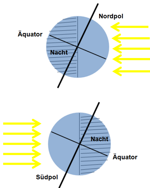
Abbildung 1: Position der Erde zur Sonne am (Nord-)Sommeranfang (oben) und am (Nord-)Winteranfang (unten)
