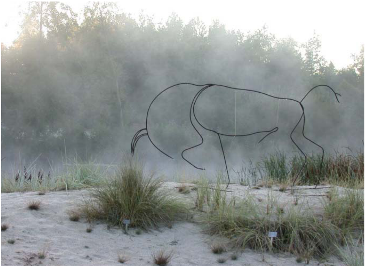
Abbildung 9: Seerauch über einem kleinen Teich im Ökologisch-Botanischen Garten der Universität Bayreuth
