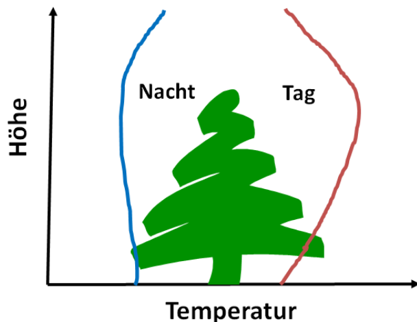
Abbildung 8: Temperaturverlauf in und über dem Wald am Tag und in der Nacht.
