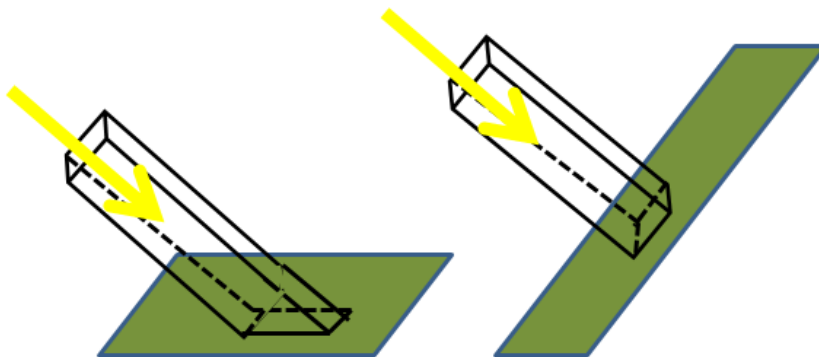
Abbildung 6: Schematische Darstellung von senkrechtem (rechts) und schrägem (links) Einfall der Sonnenstrahlen auf eine Fläche.
