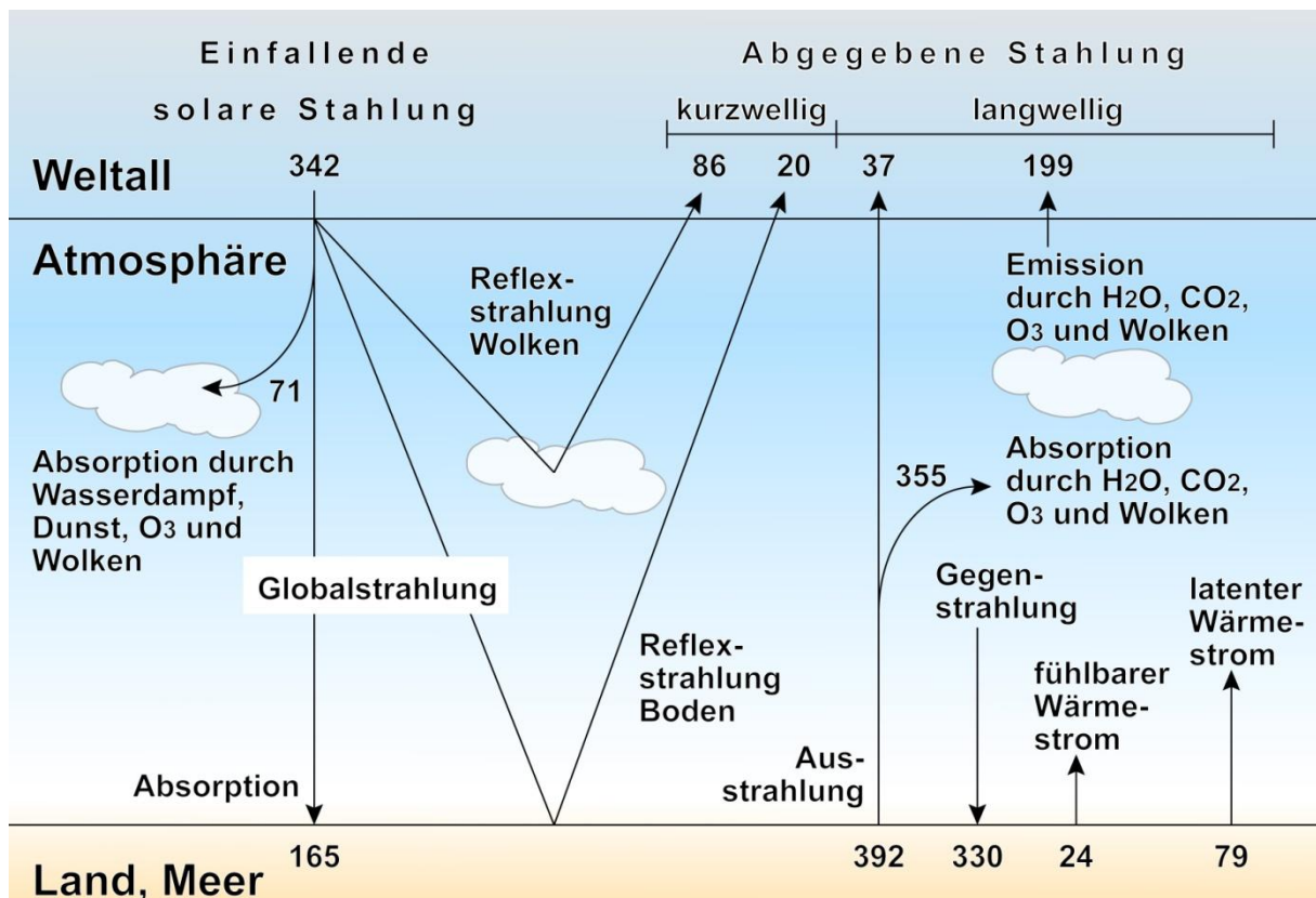
Abbildung 3: Kreislauf der Strahlungs- und Energieflüsse in der Atmosphäre (Zahlenangaben in \text{W m}^{-2} )
