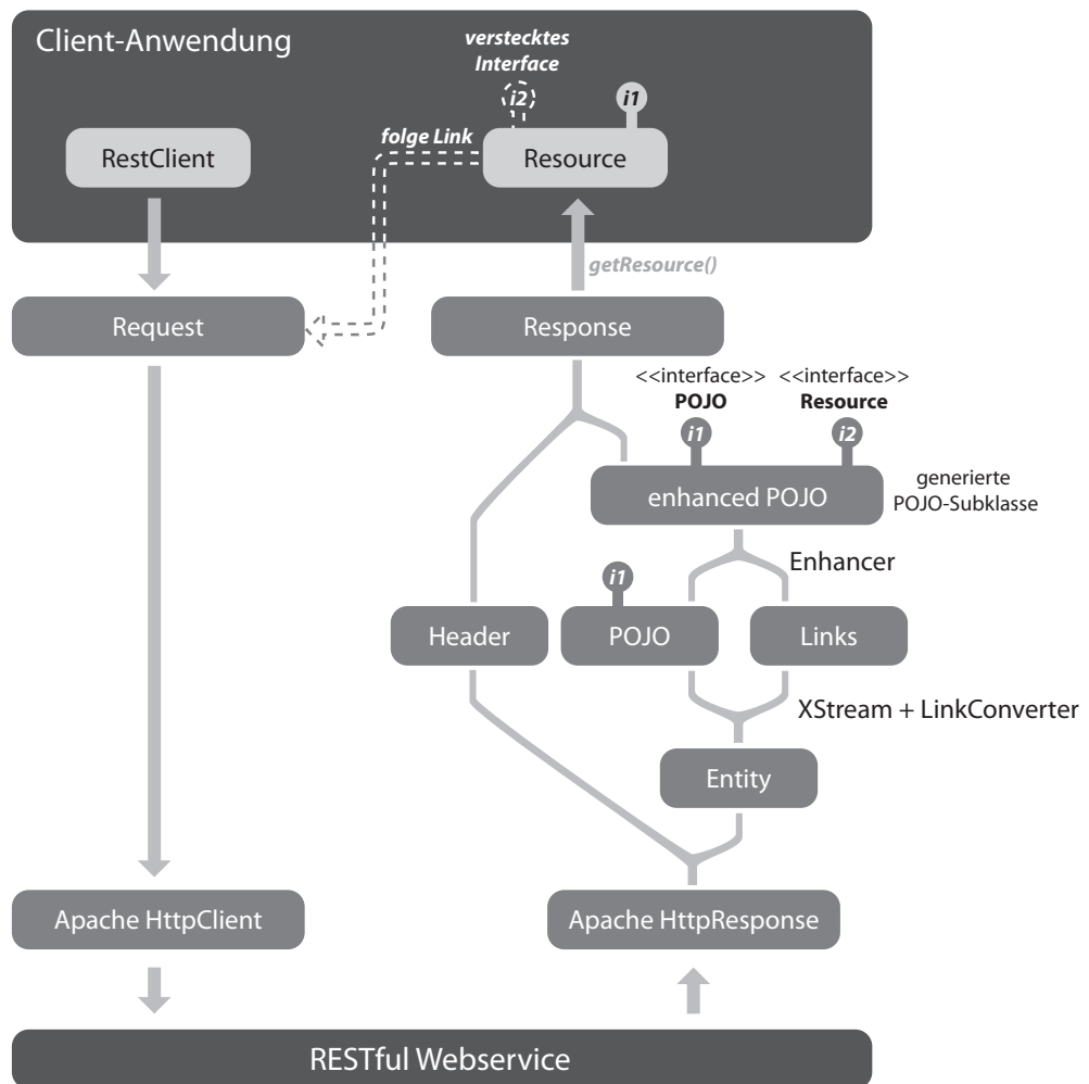
Abbildung 6: Kommunikationsablauf und Umgang mit Hypermedia im Restfulie-Framework
