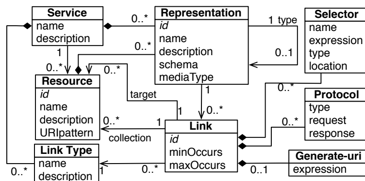
Abbildung 9: ReLL Metamodell aus [4]
