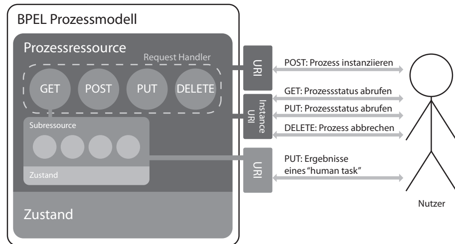
Abbildung 8: Aufbau von „BPEL for REST“-Prozessmodellen
