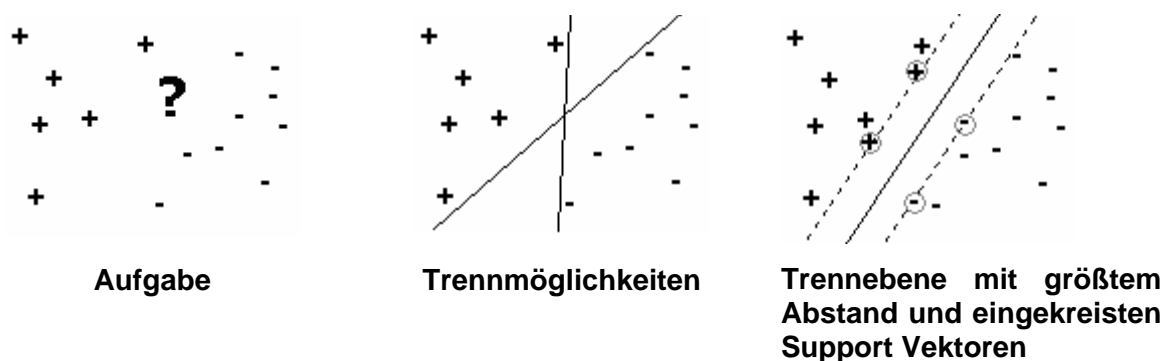
Abbildung 4.1: Binäre Klassifikationsaufgabe
