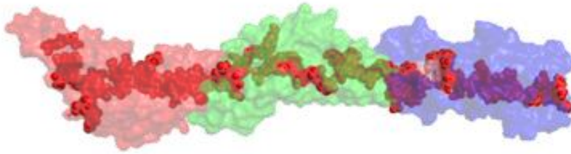
OmcZ
