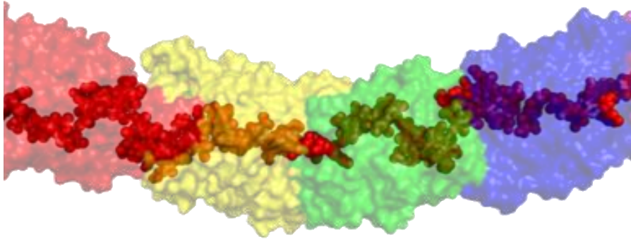
PilA
