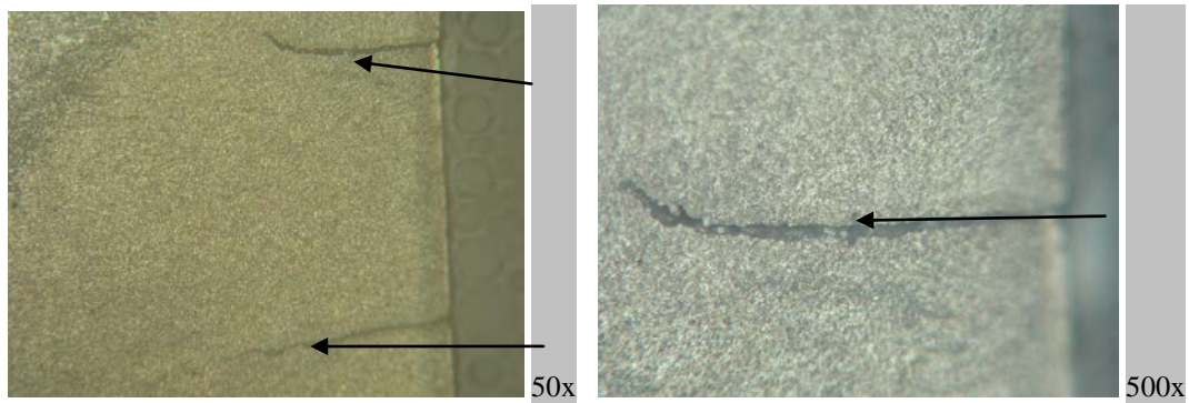
Gambar 3. Retak lainnya pada daerah HAZ halus berupa transgrannular crackings . Etsa:nital 2% dan Kalling reagent.
