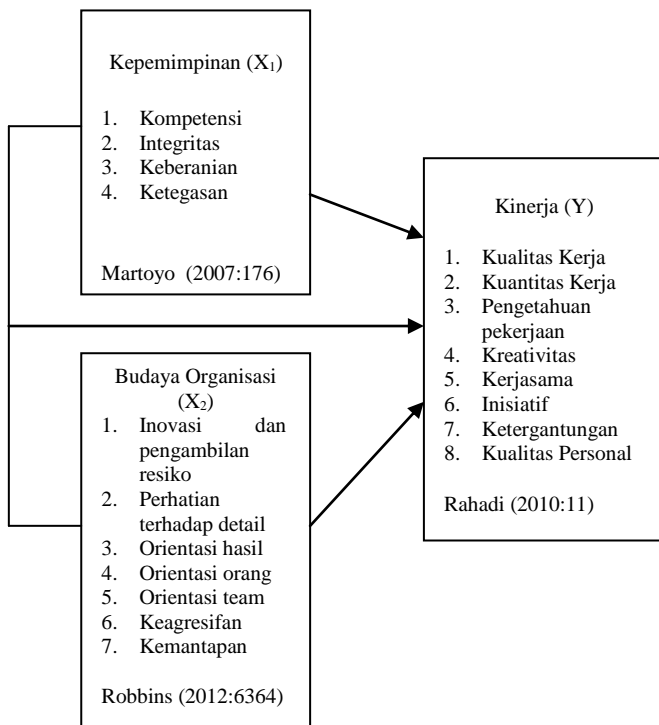
Gambar 1.1. Kerangka Pemikiran
