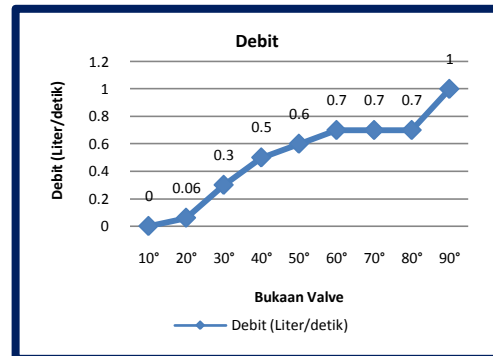
Gambar 3. Grafik Debit Air
