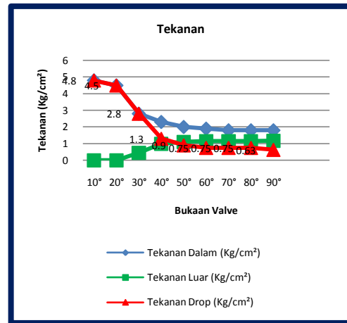
Gambar 8. Grafik Tekanan
