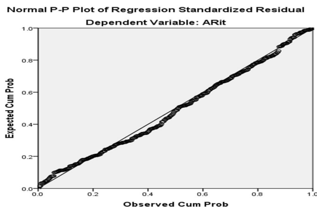
Gambar 4.2. Hasil Uji Normalitas Variabel Abnormal Return
