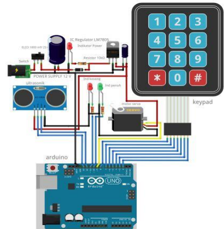
Gambar 6. Rangkaian Sistem Keseluruhan
