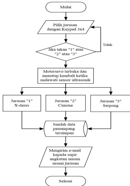
Gambar 4. Flowchart Yang Telah Diusulkan
