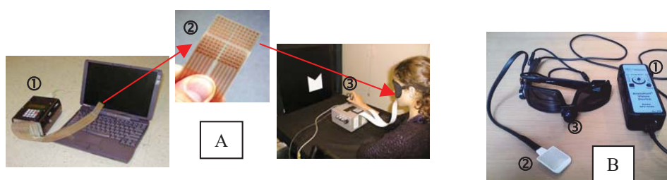
Figure 1 : Version TDU du TVSS et ses 3 composants (①interface informatique/contrôle de l'intensité de stimulation, ②matrice buccale, ③micro-caméra). A : version 1998 de Kaczmarek et Tyler ; B : version 2010 BrainPort® Vision Devive VI00 .
