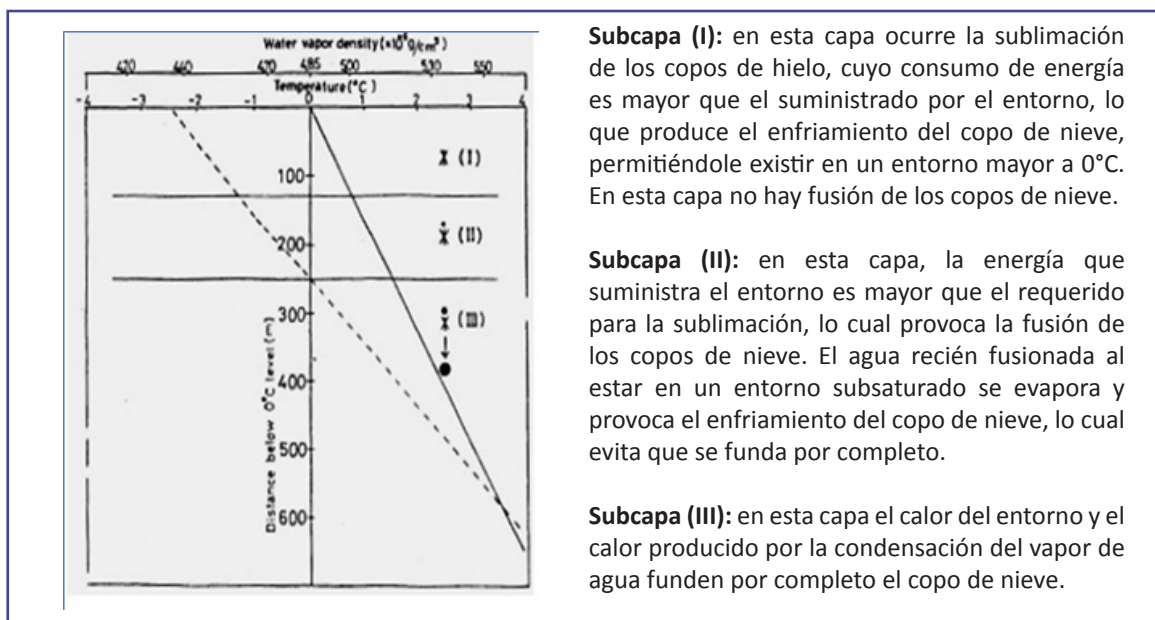
Figura 2: Esquemático de los efectos de la temperatura del aire y vapor de agua densidad del aire en la fusión de los copos de nieve por debajo del nivel de congelación. Imagen tomada de Matsuo y Sasyo (1980a)
