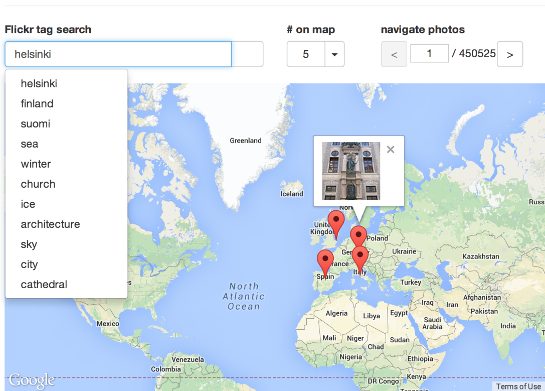
Kuva 6.1: Kuvakaappaus esimerkkisovelluksesta
