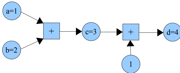
Kuva 3.1: Esimerkki riippuvuusverkosta
