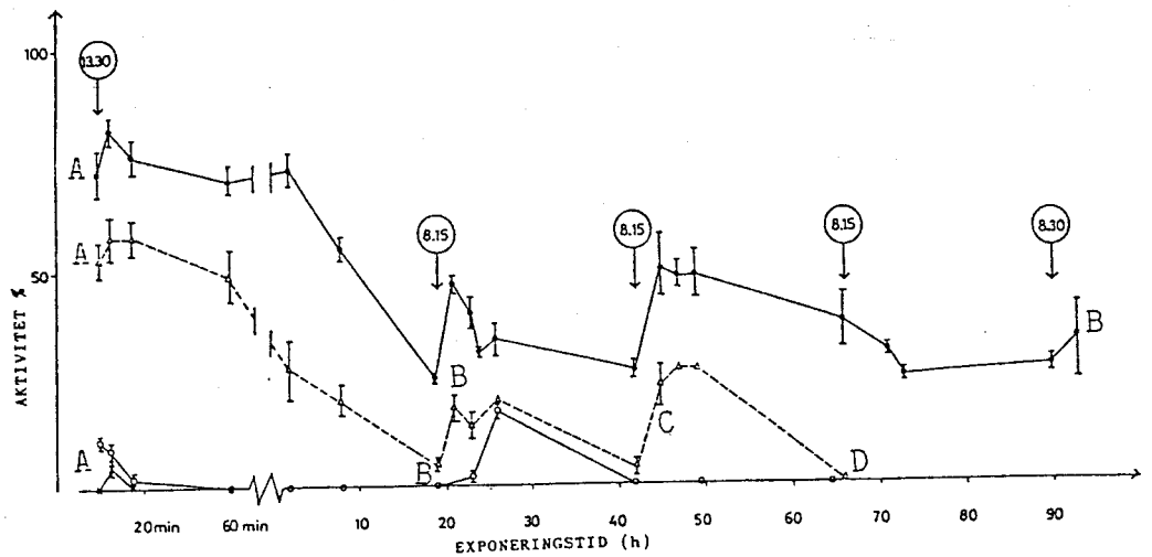
Fig. 6. Test 2. Rörelseaktiviteten hos snäckor exponerade för 0,1 % dispersant (x—), 10 % olja (Δ---) och 1/100 dispersant/olja (4 ml dispersant till 400 ml olja) (○—). Kontroll (●—). Mellan bokstäverna A-B anger värdet medeltalet hos tre akvarier, B-C medelvärdet från två akvarier och C-D värdet från ett akvarie. Dygnet's första mätning ○
