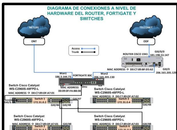
Figura 13. Diagrama de conexiones a nivel de hardware del router, fortigate y switches.
