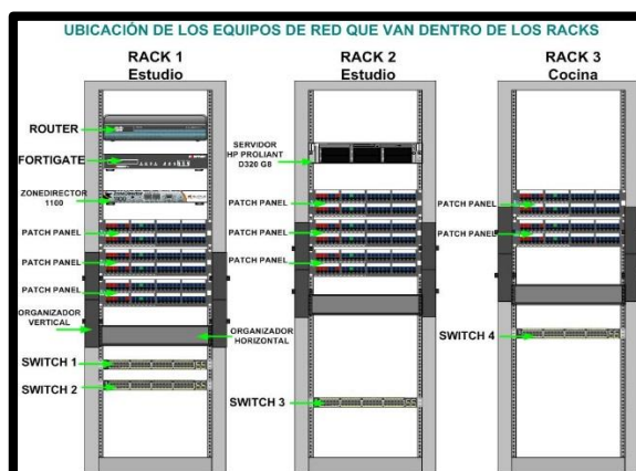
Figura 15. Ubicación de los equipos de red que van dentro de los Racks.
