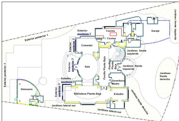
Figura 5. Vista general de la planta baja de la vivienda.
