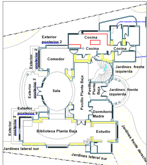
Figura 7. Planta baja de la vivienda parte central.
