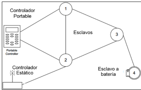
Figura 2. Diagrama básico de una red Z-Wave.
