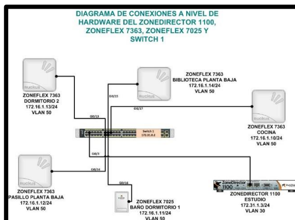
Figura 14. Diagrama de conexiones a nivel de hardware del Zonedirector 1100, zoneflex 7363, zoneflex 7025 y switch 1.
