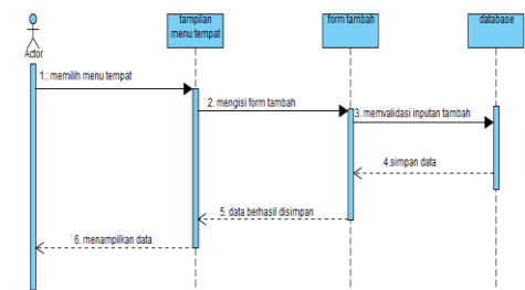
Gambar 7. Sequence Diagram Tambah Data Tempat
