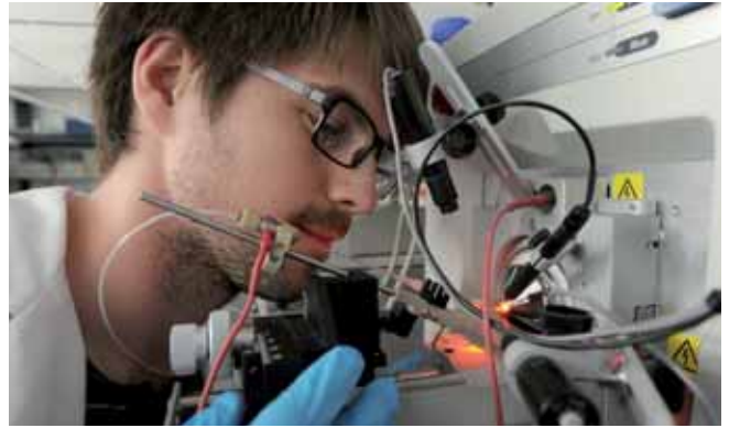
Bereits geringe Proteinmengen können identifiziert und quantifiziert werden: Ein Wissenschaftler am MDC justiert die Position der Nano-HPLC-Säule. Diese fraktioniert die Peptide, bevor sie im Massenspektrometer gemessen werden. Foto: MDC/D. Ausserhofer
