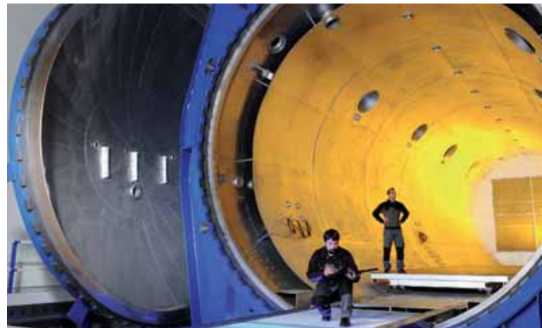
Der größte Forschungsautoklav der Welt steht im DLR Stade. Mit ihm härten die Wissenschaftler Flugzeugbauteile aus kohlestofffaserverstärktem Kunststoff (CFK) aus. BALU (Biggest Autoclave Laboratory Unit) wurde 2012 in Betrieb genommen und ist 20 Meter lang bei einem Durchmesser von nahezu sechs Metern. Foto: DLR
