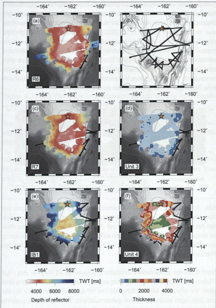
Abb. 2: Bathymetrische Karte des High Plateaus, Subplateau des Manihiki Plateaus, überlagert mit den reflexionsseismischen Profilen von Expedition SO224 (b) und DSDP Leg 33 Site 317 Bohrloch (orangener Stern). Die Reflektortiefen von R6 (a), R7 (c) und IB1 (e) zeigen deutliche Erhöhung im Zentrum des Plateaus. Schichtdicken von Unit 3 (R6-R7), sowie Unit 4 (R7-IB1) zeigen starken Vulkanismus während der Hauptphase (f) und eine Phase mit weniger Vulkanismus während der späteren Phase (d).
