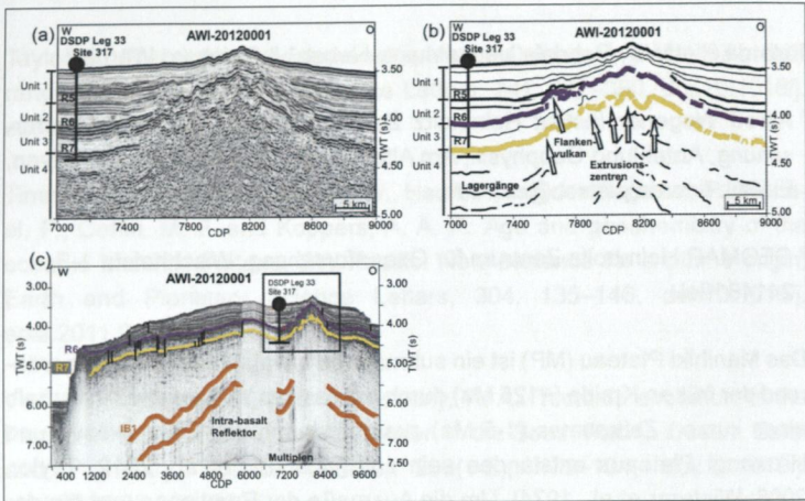
Abb. 1: Das Ost-West verlaufende Profil AWI-20120001 kreuzt das DSDP Leg 33 Site 317 Bohrloch bei CDP 7100. Es zeigt die reflexionsseismische Stratigraphie (a, c) und Interpretation (b). Hervorgehoben sind die Reflektoren R7 (gelb) und R6 (violett), die mit dem Ende der Hauptphase bzw. der späten Phase korrelieren, sowie den intrabasaltischen Reflektors IB1 (orange).
