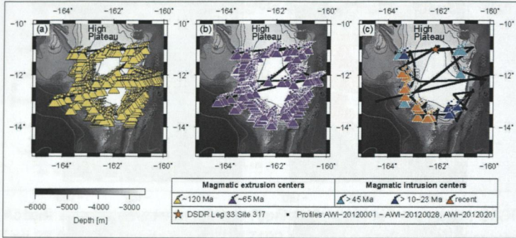
Abb. 3: Verteilung der kartierten extrusiven und intrusiven Strukturen auf dem High Plateau, Subplateau des Manihiki Plateaus. Die Extrusionszentren der (a) Hauptphase, assoziiert mit Reflektor R7 und (b) späteren Phase assoziiert mit Reflektor R6 zeigen eine Verlagerung vom Zentrum hin zu den Flanken. Intrusive Strukturen (c) vorallem im südwestlichen Teil des Plateaus vorhanden.
