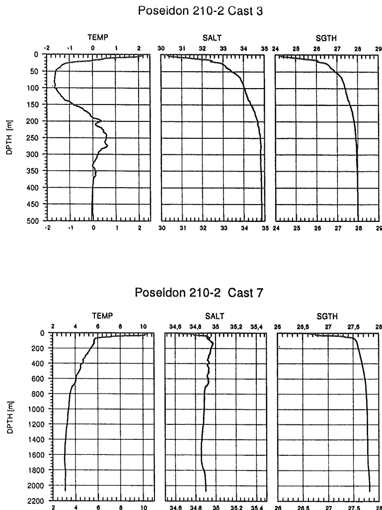
Abb. 25: CTD Profile "POSEIDON"- Reise 210/2 als Beispiel für die Hydrographie in der Dänemarkstraße: a) Tiefenprofil des kalten Ostgrönlandstroms, b) Tiefenprofil des relativ warmen Irmingerstroms.
