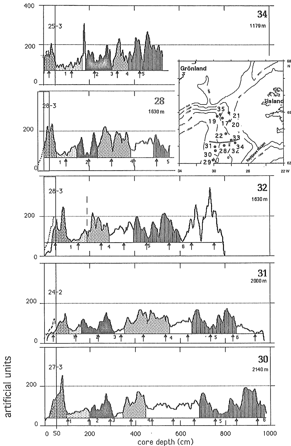
Abb. 21: Vorläufige stratigraphische Korrelation der südlichen Kerne nach den Kurven der magnetischen Suszeptibilität. Pfeile markieren die Lage der Kern-Schnitte, gestrichelt sind die Kurven aus den entsprechenden GKG-Profilen.
