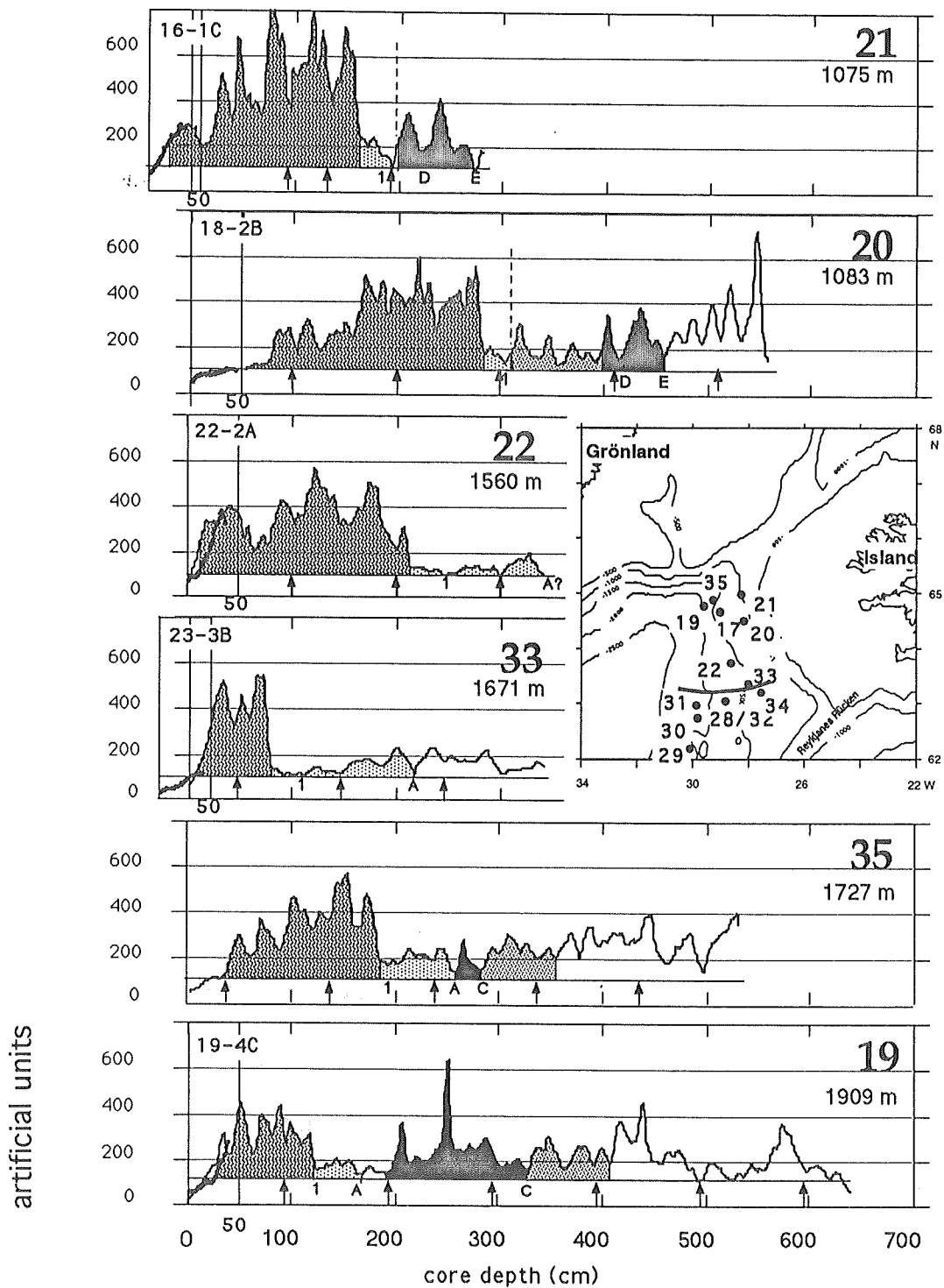
Abb. 22: Vorläufige stratigraphische Korrelation der nördlichen Kerne nach den Kurven der magnetischen Suszeptibilität. Pfeile markieren die Lage der Kern-Schnitte, dick ausgeführt sind die Kurven aus den entsprechenden GKG-Profilen.
