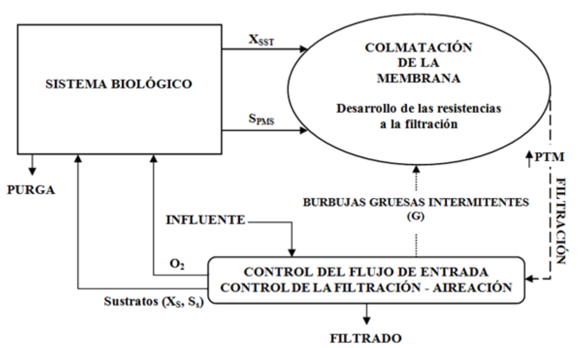
Fig. 3. Esquema conceptual del modelo desarrollado por Zarragoitia, considerando todas las partes integrantes del sistema ( S_{PMS} Concentración de productos microbianos solubles; X_S Concentración de sustrato lentamente biodegradable y S_S Concentración de sustancias orgánicas fácilmente biodegradables). 31
