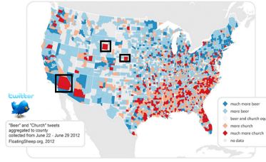
Fig. 2: Twitter Anomalies
