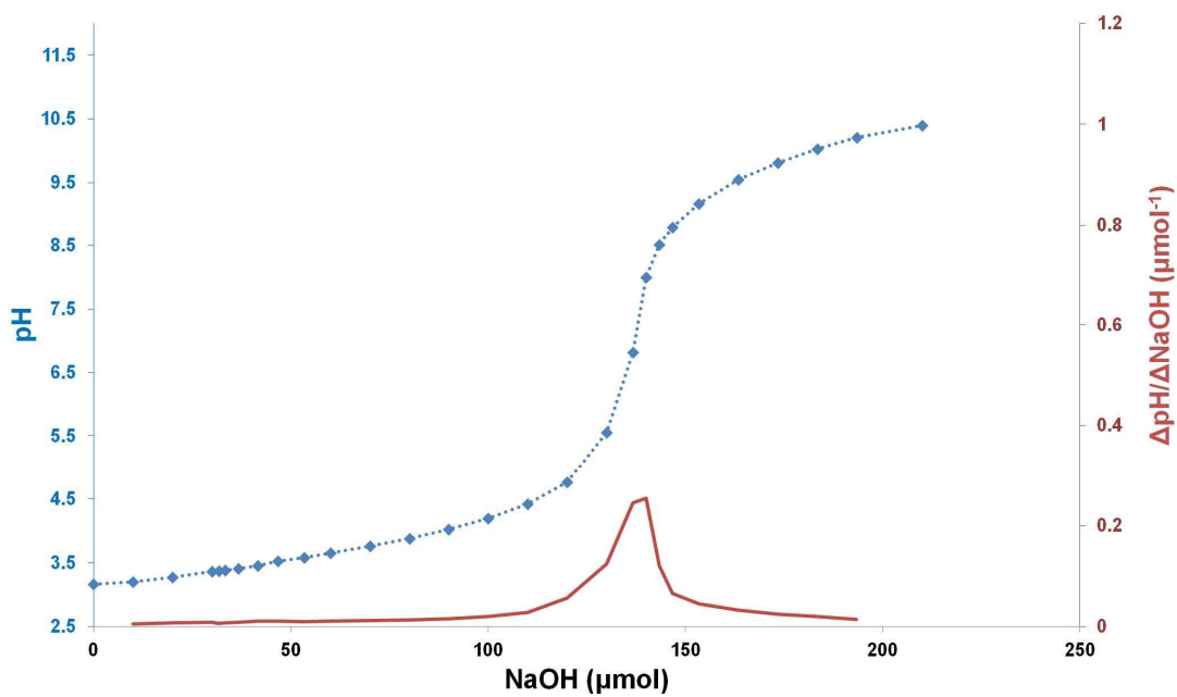
Fig. VI.8. Acid titration for mPEG 2000 COOH -♦- pH, — \Delta\text{pH}/\Delta\text{NaOH}
