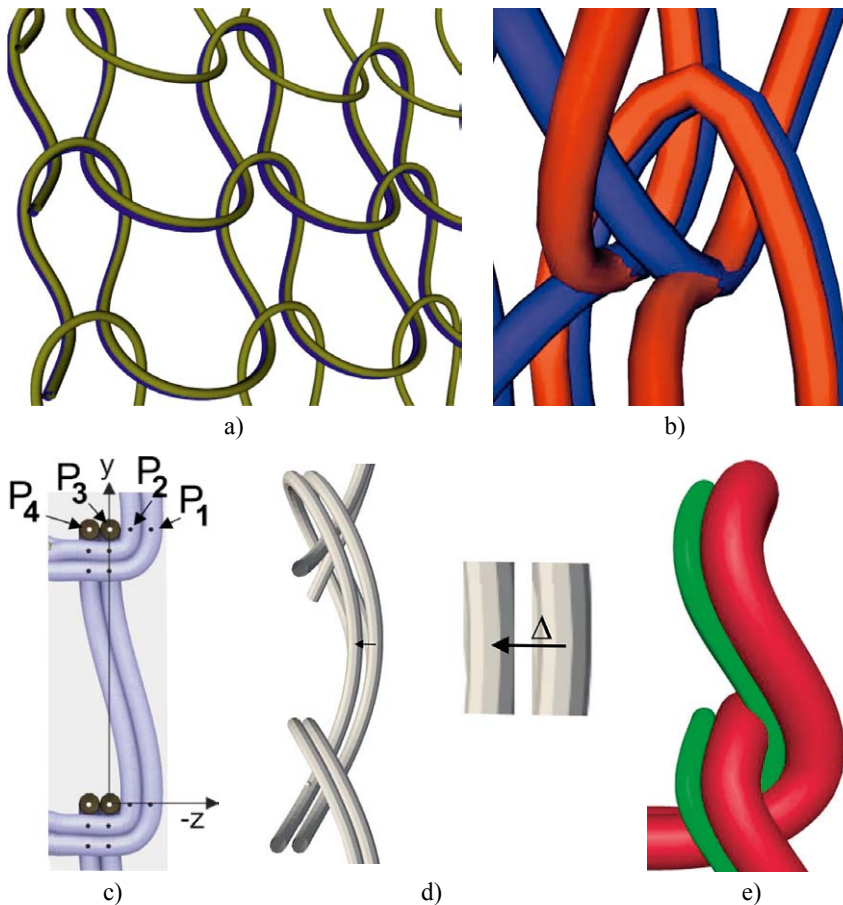
S1.3 Primjeri osnovnih parametara pri 3D modeliranju strukture platiranih pletiva:
