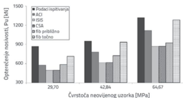
Slika 18. Usporedba rezultata ispitivanja i teorijske nosivosti CFRP-a
