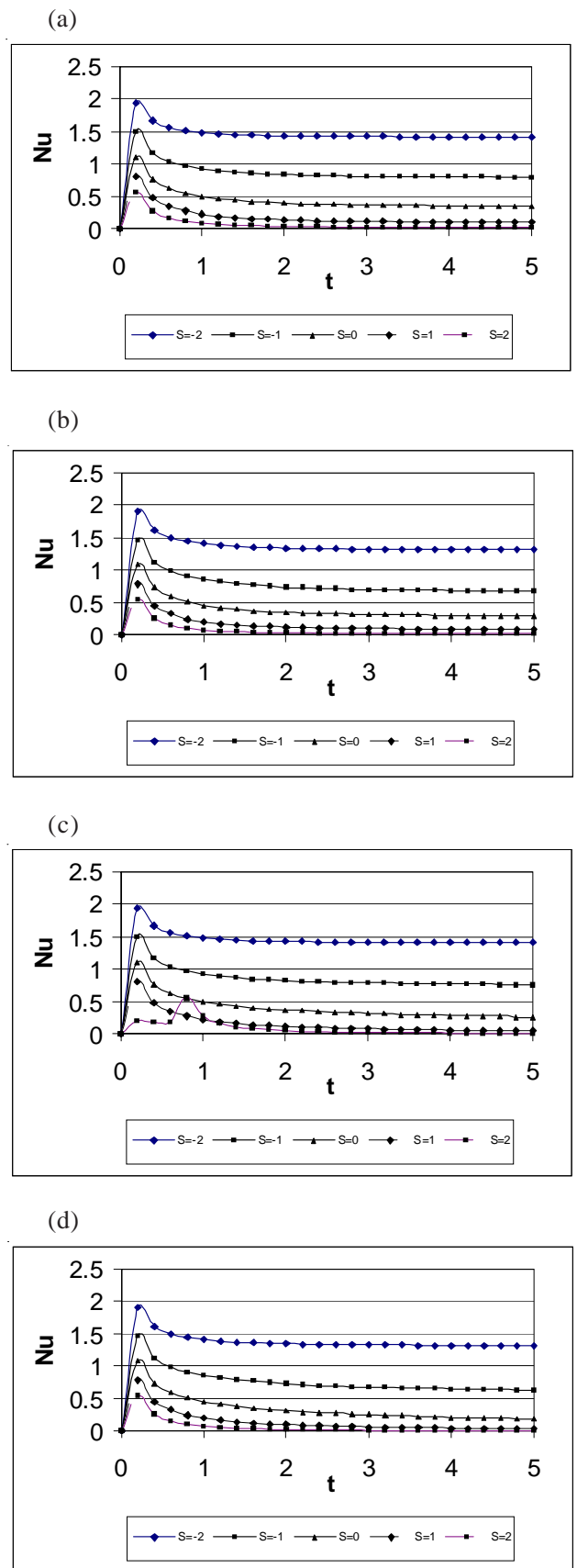
Fig. 2 Time development of the Nusselt number Nu_u : (a) K=0, M=0 ; (b) K=1, M=0 ; (c) K=0, M=1 ; (d) K=1, M=1
