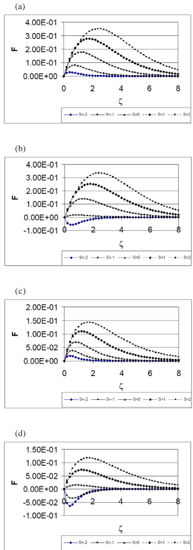
Fig. 4 The radial velocity profile vs. S : (a) K=0, M=0 ; (b) K=0.5, M=0 ; (c) K=0, M=1 ; (d) K=0.5, M=1
