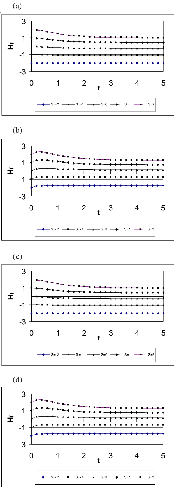
Fig. 1 Time development of the axial velocity at infinity H_f : (a) K=0, M=0 ; (b) K=1, M=0 ; (c) K=0, M=1 ; (d) K=1, M=1
