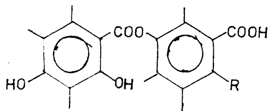
Rajah 1. Formula struktur asas bagi kelas utama depsida.
