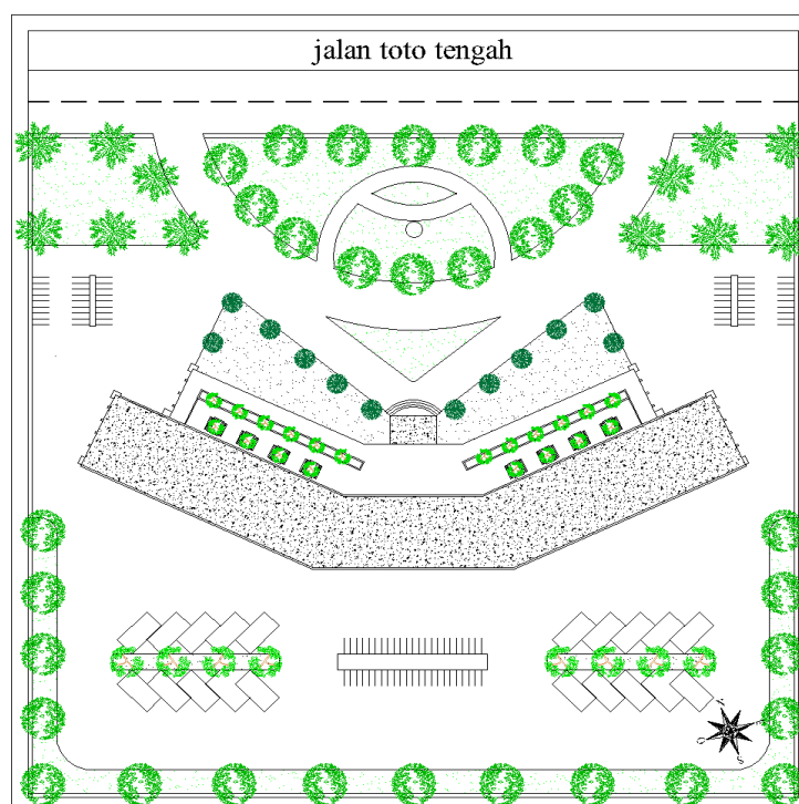
Gambar Layout Bangunan
